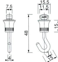
CAフック
