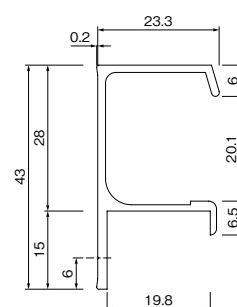
断面図
