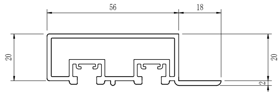
上レール
