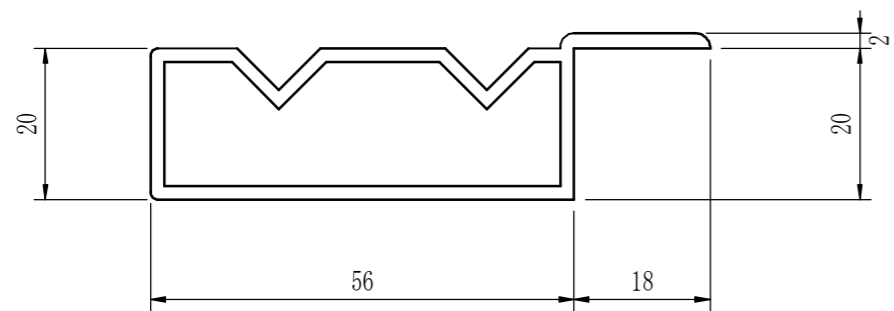
したレール
