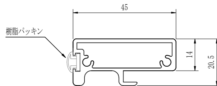
扉縦枠
