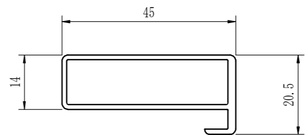
扉横枠
