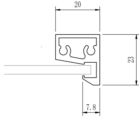
枠断面図
